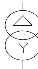
Pašpatēriņa transformators 10/0,4kV - 25kVA
